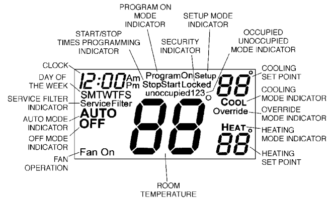
Fig. 1 — Thermostat Display
