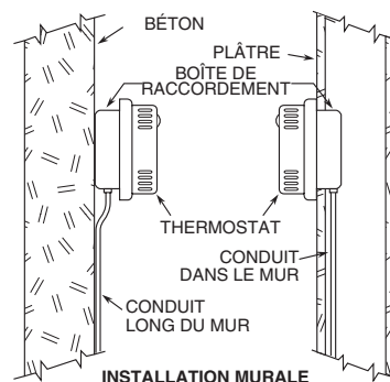
La plaque de montage du thermostat est dotée de deux trous séparés par 3/16" qui servent à fixer la commande sur une boîte de raccordement ordinaire.
