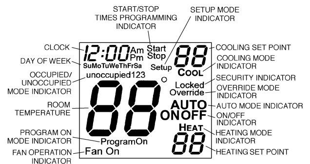
Fig. 1 — Thermostat Display
